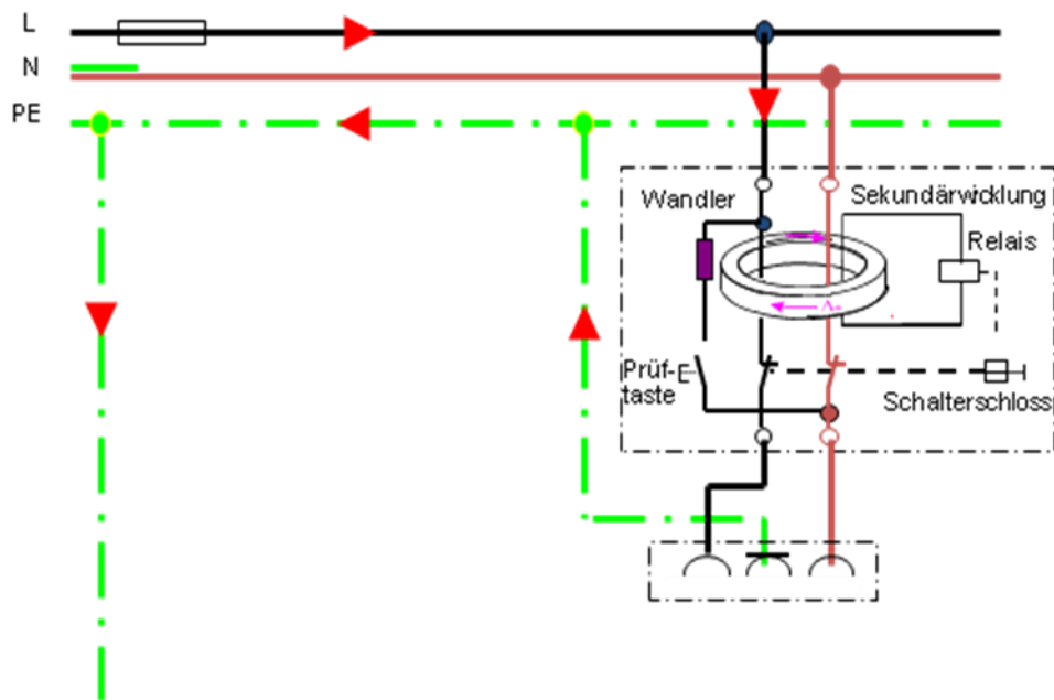
Abb. 27: Funktion einer Fehlerstrom-Schutteinrichtung (RCD)
