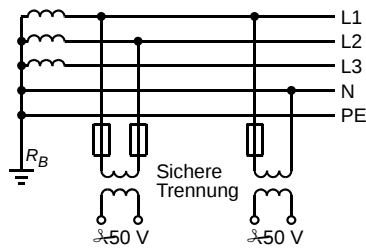
Abb. 24: SELV
