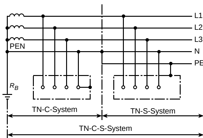
Abb. 15: a) TN-C-S-System
